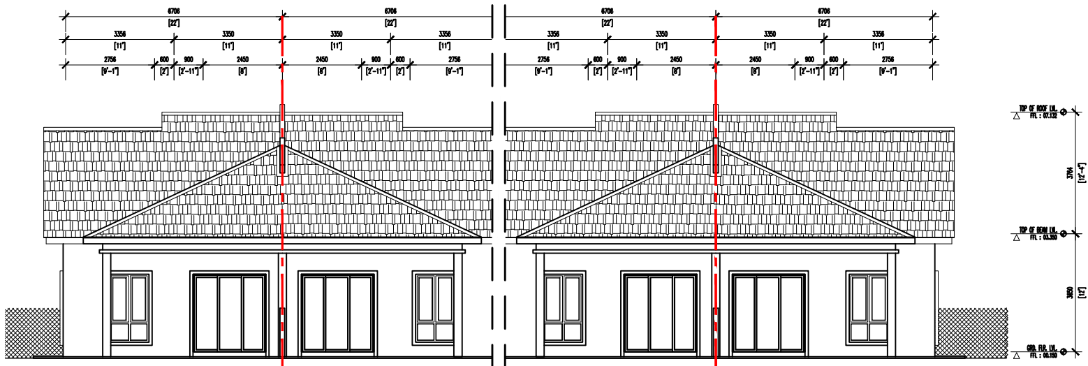
FRONT ELEVATION SKALA : 1 : 1 0 0
