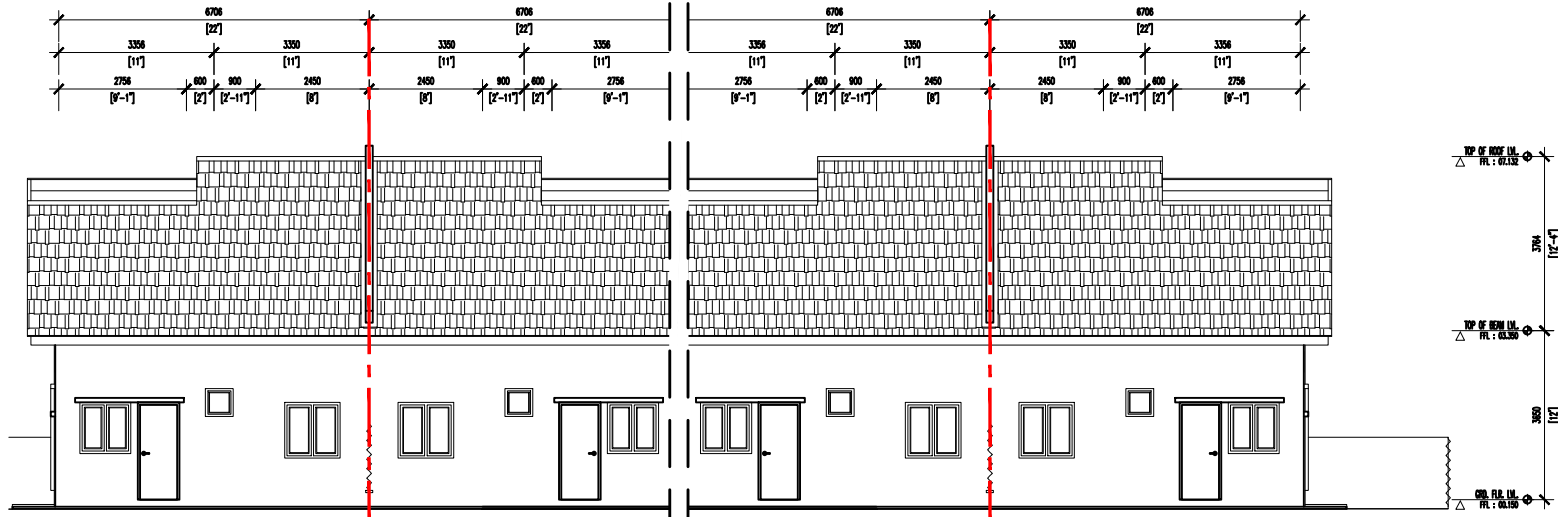
REAR ELEVATION SKALA : 1 : 1 0 0
