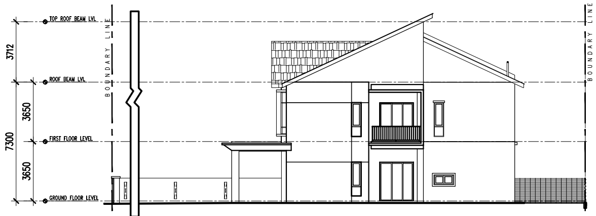
RIGHT ELEVATION
